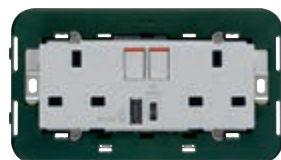
■ 14224.AC.SL SICURY 2P+E 13 А 250 В~ с двумя выключателями 2Р, выхо- дом USB типа А и выходом USB типа С. Глубина: Глубина: 21 мм
