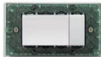
Δ 14450.SL Устройство чтения/программирования карт-транспондеров в настольной коробке 4 модуля. Укомплектовывается накладкой 4 модуля. Размеры: 142,5x78,4x9x89,2 мм
