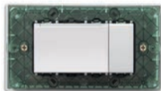
14450 Устройство чтения/программирования карт-транспондеров в настольной коробке 4 модуля. Укомплектовывается накладкой 4 модуля. Размеры: 142,5x78,4x9x89,2 мм
