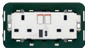
■ 14224.AC SICURY 2P+E 13 А 250 В~ с двумя выключателями 2Р, выхо- дом USB типа А и выходом USB типа С. Глубина: Глубина: 21 мм
