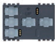
21457 Считыватель транспондерных карт Eikon Tactil, стандарт KNX, 2 HP релейных выхода 4 А 24 В~, 2 входа, 12-24 В~ 50/60 Гц и 12-24 В пост. тока (SELV) - 3 модуля. Поставляется без транспондерной карты. Глубина: 36,5 мм
