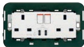
▲ 14224.CC SICURY 2P+E 13 А 250 В~ с двумя выключателями 2Р, выходом USB типа С. Глубина: Глубина: 22,8 мм
